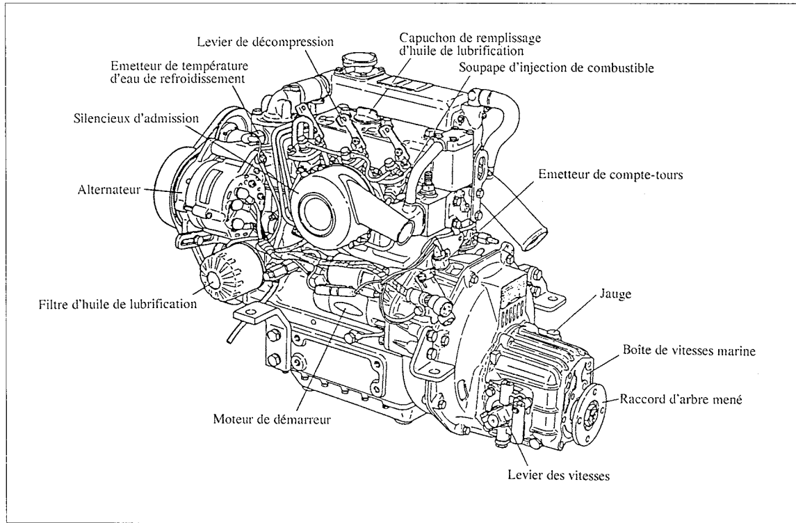
Côté admission du 3GM30F
