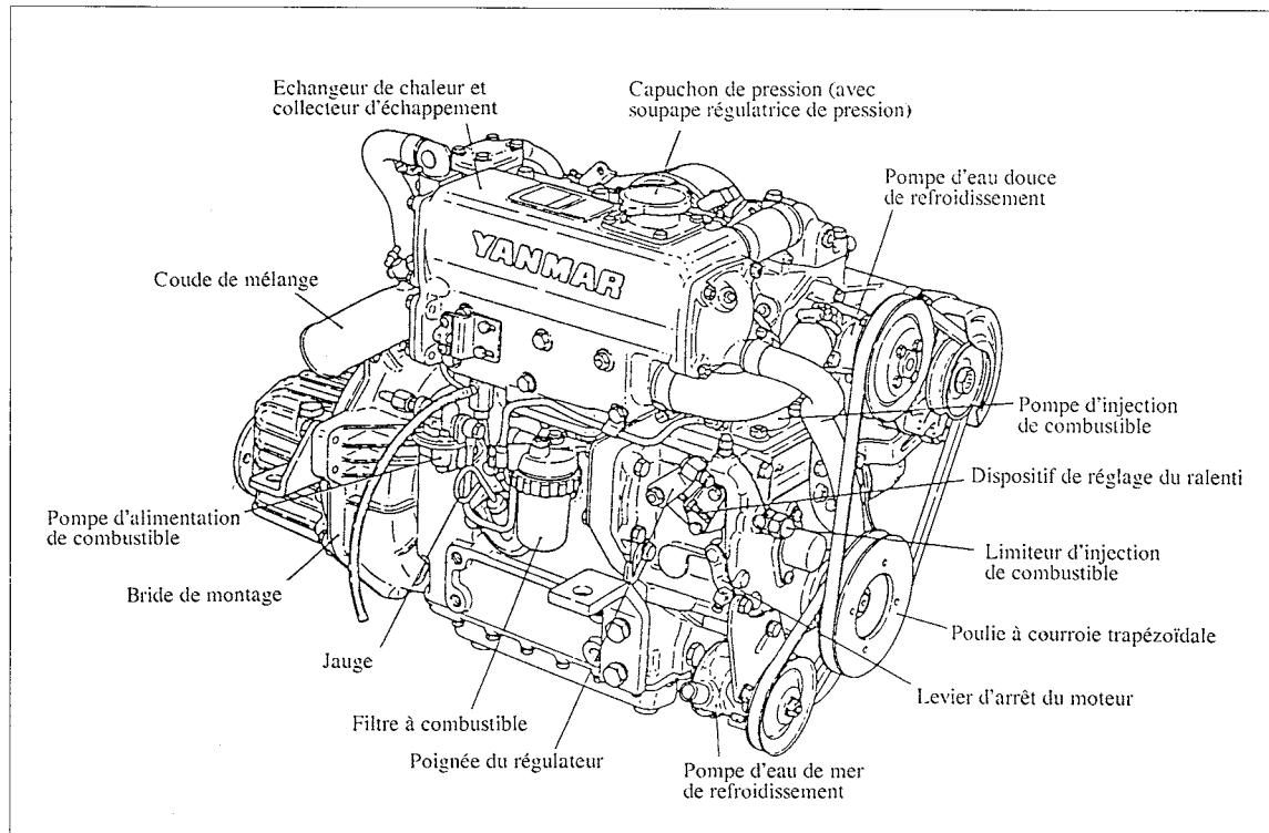
Côté échappement du 3GM30F
